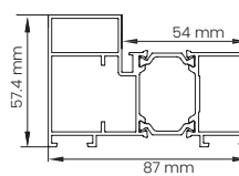
Profil ościeznicy ALU/90
