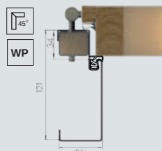
alumiowy ALU 15/54
