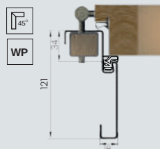
alumiowy ALU 11/54
