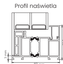
Profil naświetla
