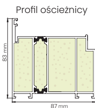
Profil ościeżnicy
