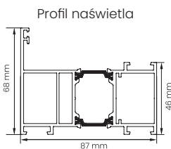
Profil naświetla
