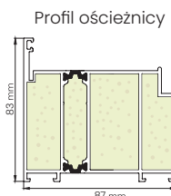
Profil ościeżnicy
