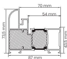
Profil ościeznicy ALU/90
