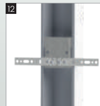
Elementy wzmacniające konstrukcję ościeznicy z kotwami montażowymi Ościeznica 15/54
