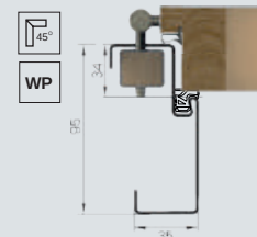
alumiowy ALU 10/54
