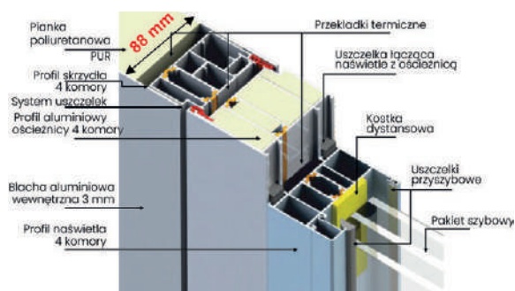
Profil ościeżnicy
