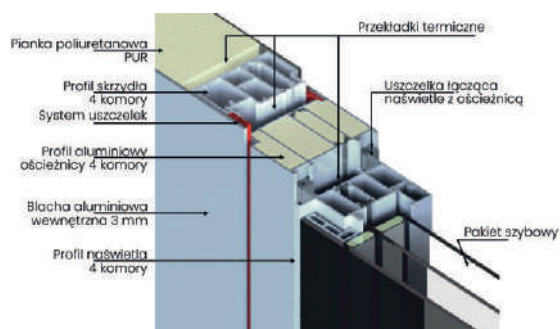
Profil ościeżnicy
